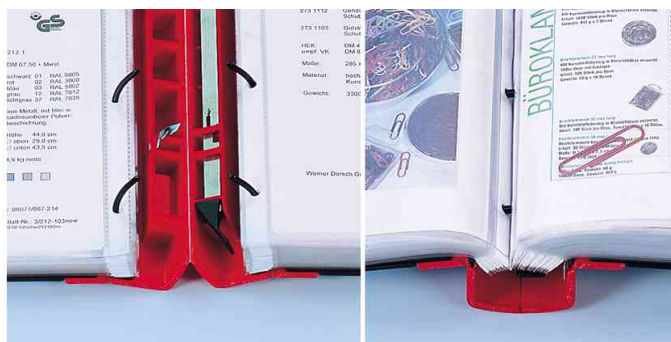
mécanisme 4 anneaux ouvert & fermé
